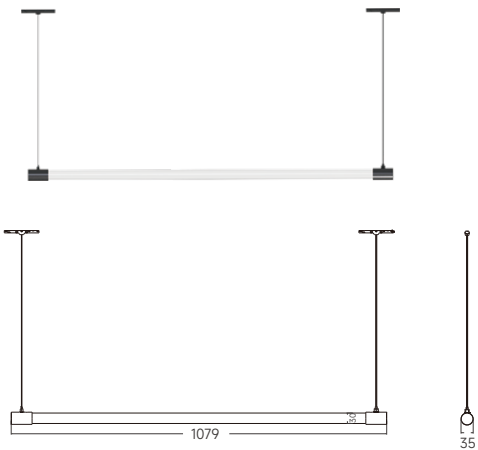
LX11-NHP10
