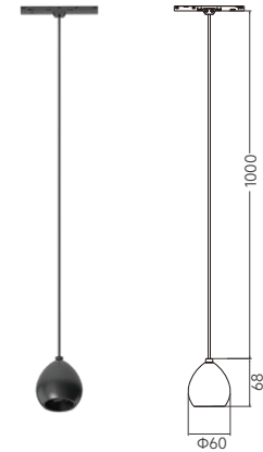
LX11-SURI 60
