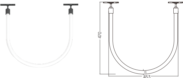
LX11-NHU12
