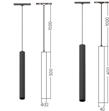
LX11-PS30/LX11-PS40
