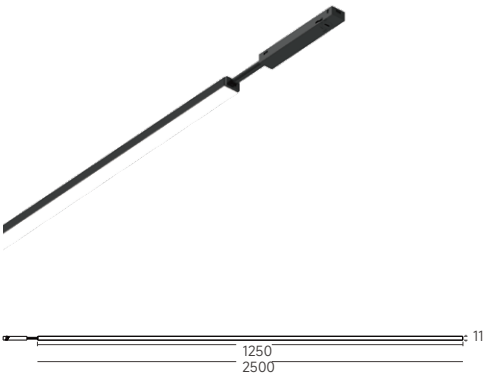
LX11-GL1250-13W LX11-GL2500-25W
