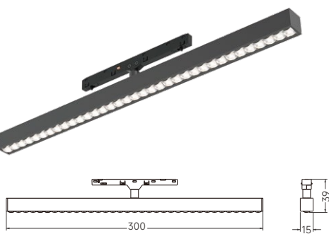
LX11-A-AL300
